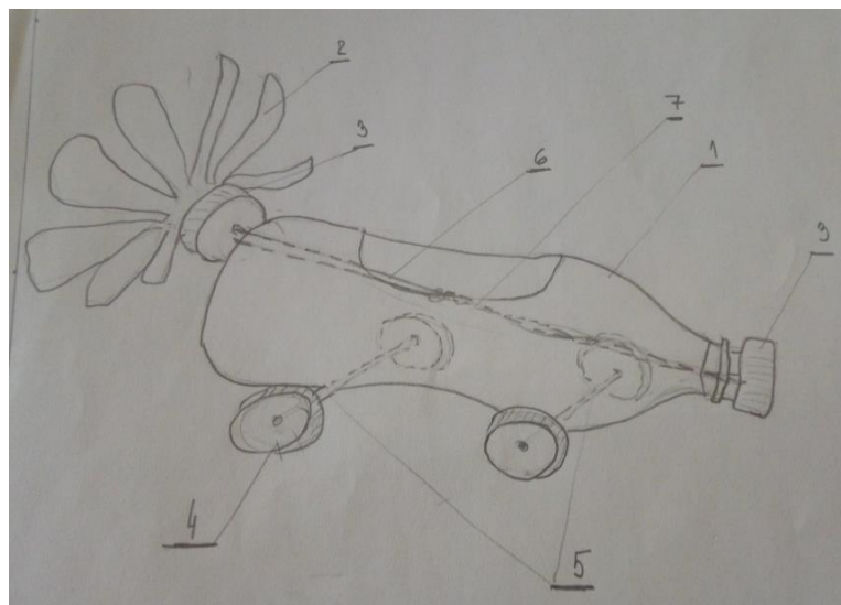
Slika 2: SESTAVNA RISBA
